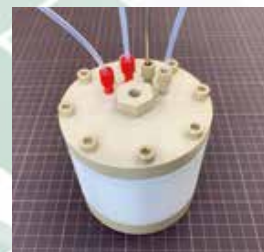
CSTR組立品(PTFE、PEEK)
