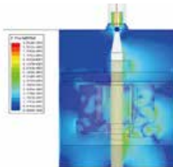
CSTR本体に水を満たした状態の同軸チャンパー内電界分布
